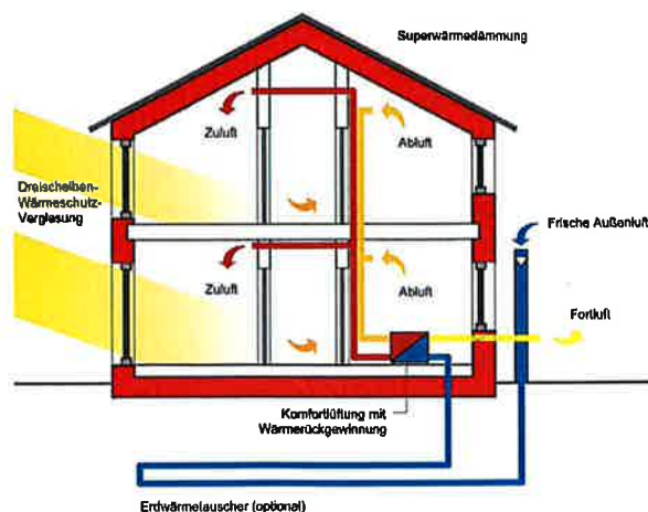
Passivhauskonzept
