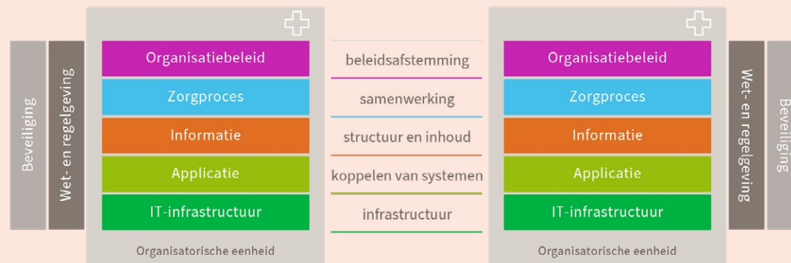
Figuur: Nictiz-vijflagenmodel
